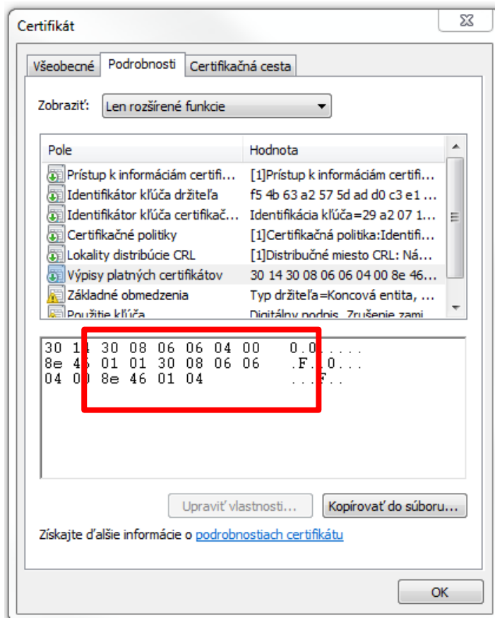
Obr. 8 - Zistenie príznaku QcSSCD v podrobnostiach certifikátu .cer
